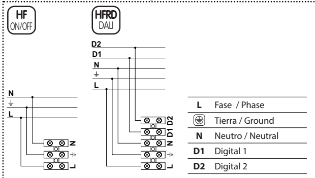
Esquema eléctrico Electric diagram
