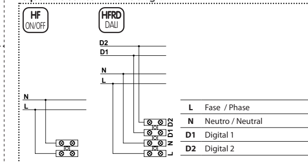
Esquema eléctrico Electric diagram
